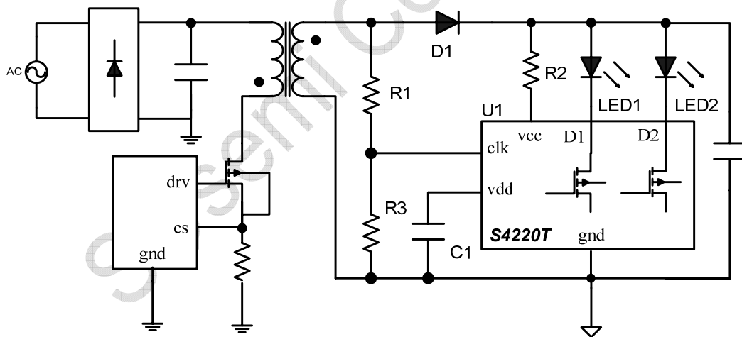
图1 S4220T的典型应用图
