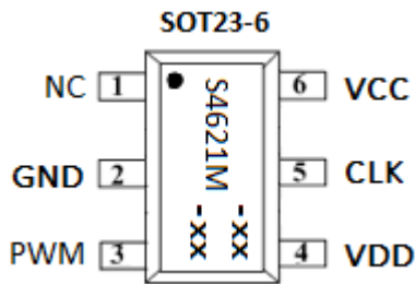
图2 脚位图
