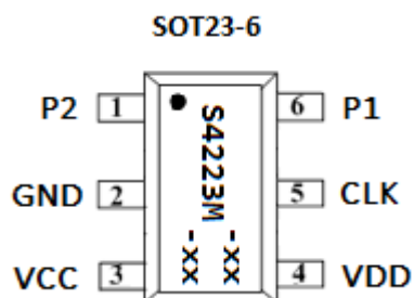
图2 脚位图
